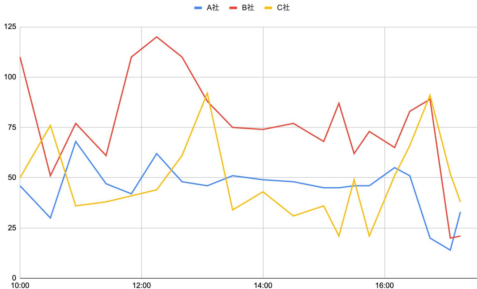
4G(LTE) ダウンロード速度推移 Mbps
