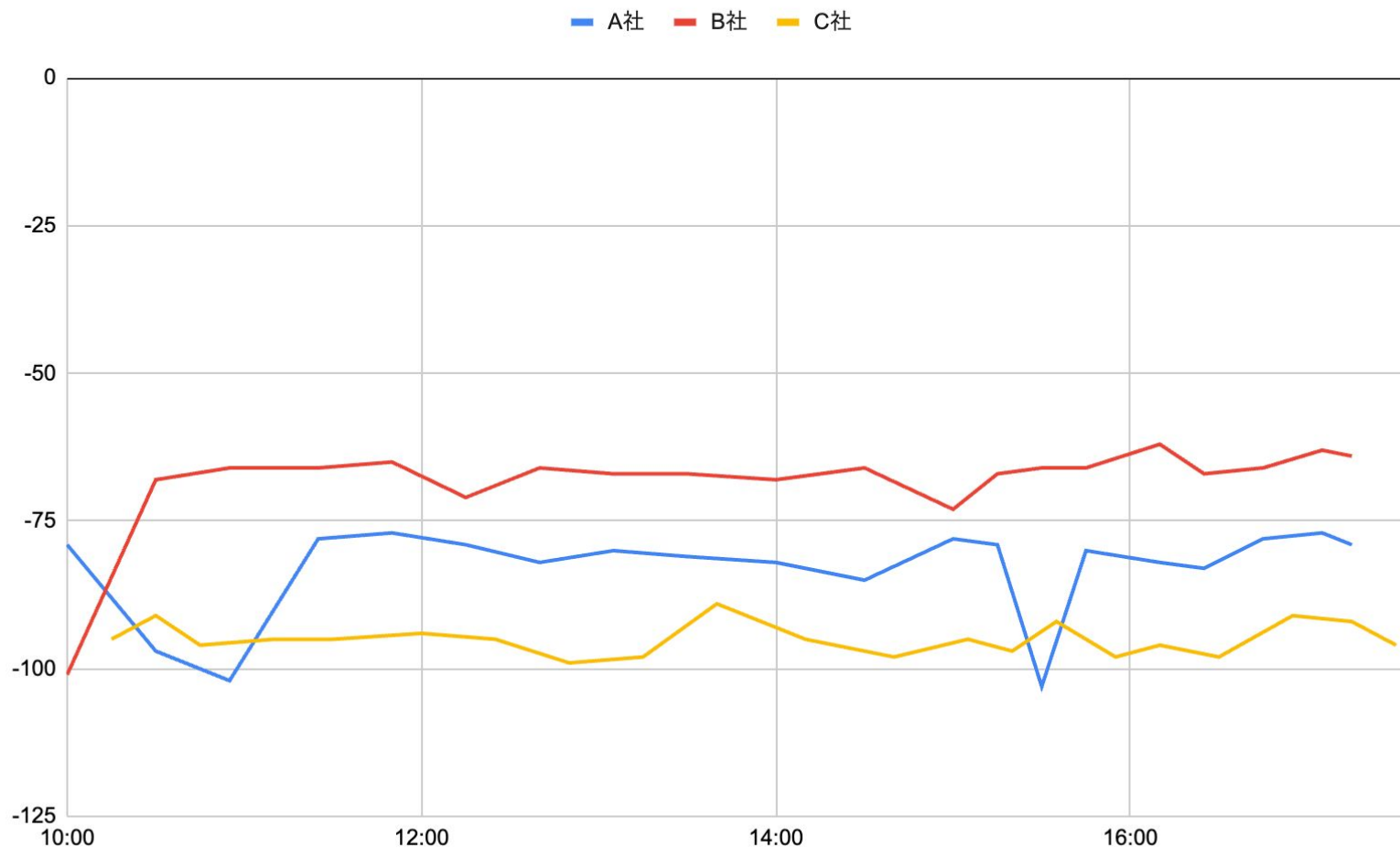
4G(LTE) RSRP推移 dBm
